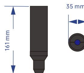
20A/30A/20E/30E隔离器输出头
