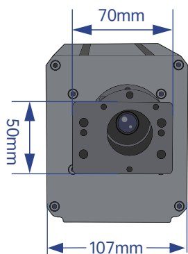
20G/30G 设备正面
