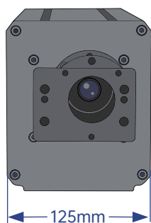
50G 设备正面
