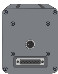
50G 设备背面
