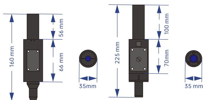
50w/60w隔离器输出头
